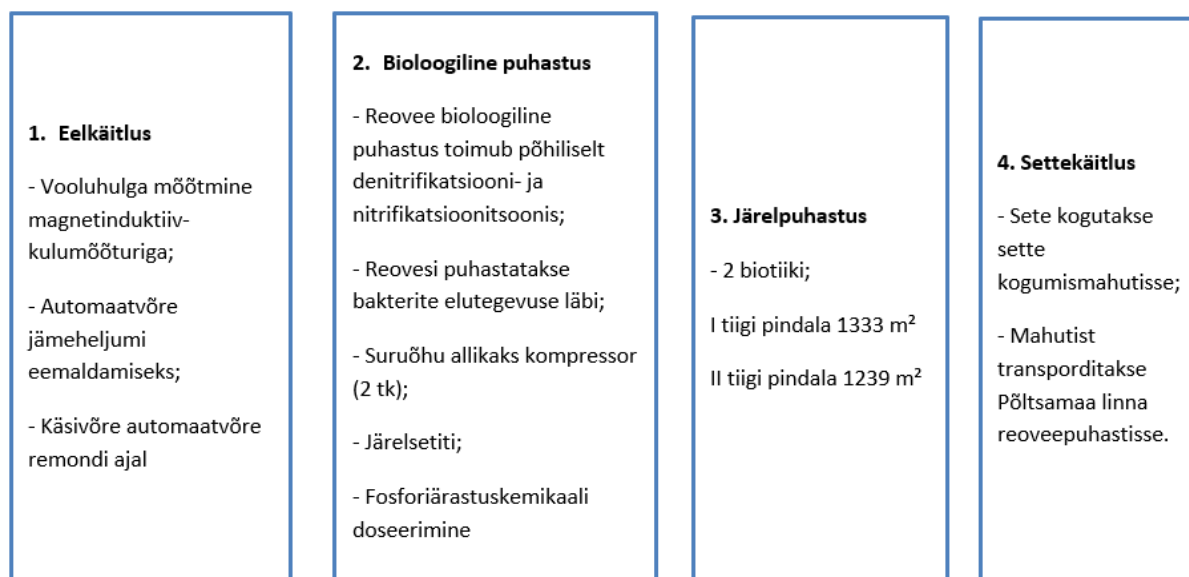
Joonis 5.1. Kolga-Jaani reoveepuhasti reoveepuhastussüsteemi etapid.
