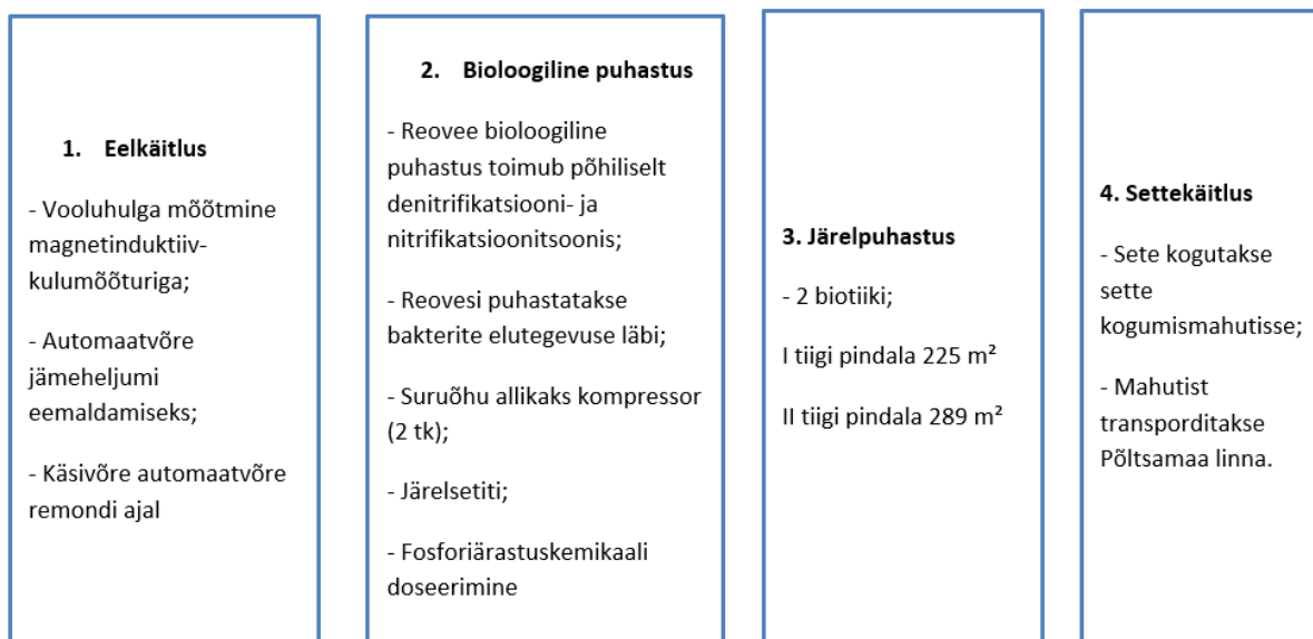
Joonis 5.2. Leie reoveepuhasti puhastusprotsessi skeem
