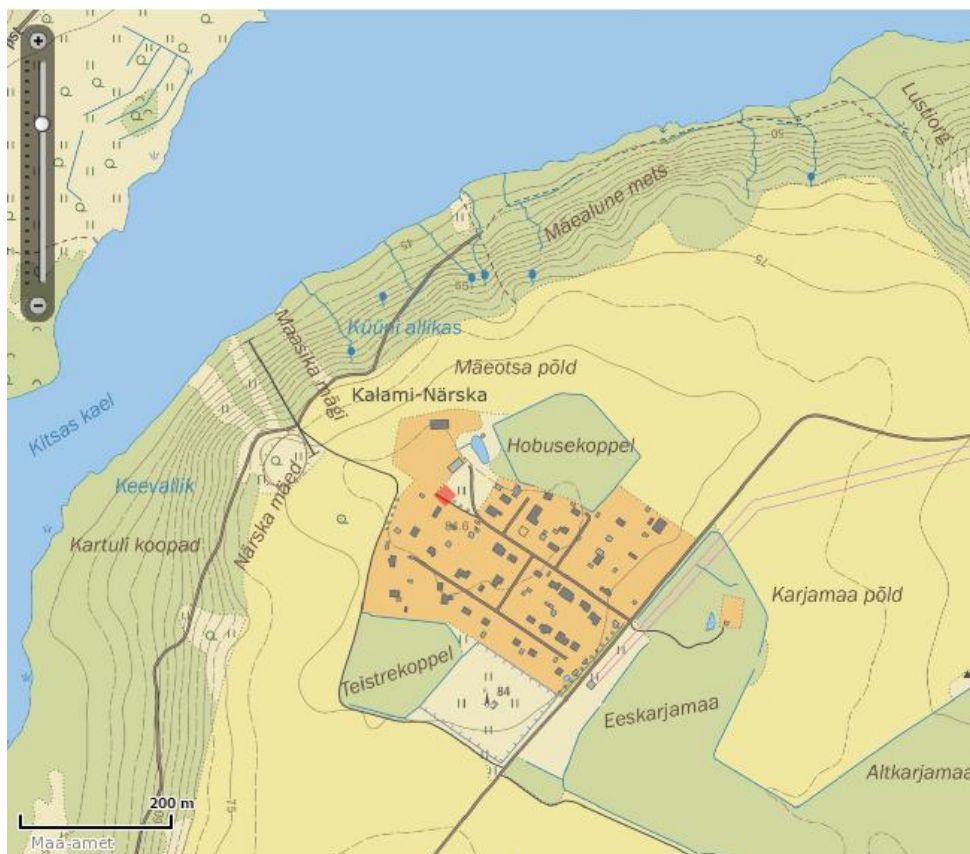
Joonis 5.1. Sakala suvilapiirkonna puurkaevpumpka kat. nr. 6030 asukoht. Allikas: Keskkonnaregister
